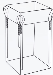
SKIRT EN GESLOTEN BODEM
